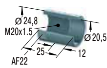
限位套筒
