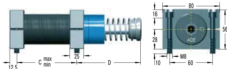
侧角支架安装
