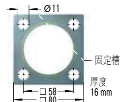
方型法兰
