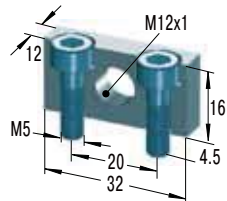
安装支架
