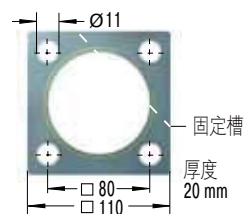
方型法兰
