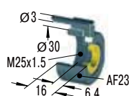
气流阀
