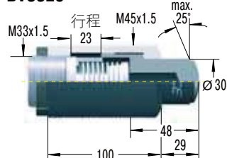
偏心转接器
