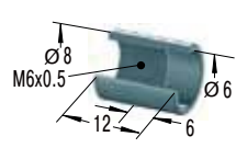
限位套筒
