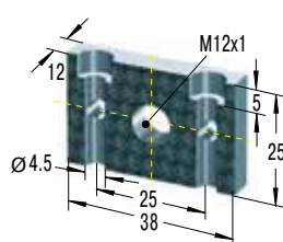
通用转接件
