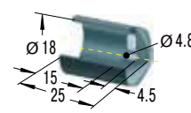
钢套
