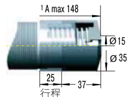
钢套
