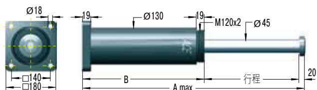
后法兰 -R
