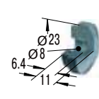
钢套
