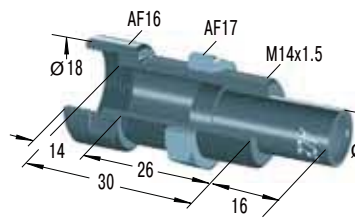
偏心转接器
