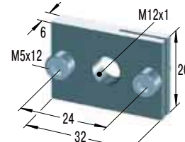
矩形法兰
