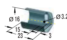
钢套
