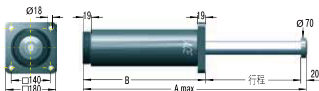
前法兰 -F
