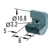
钢冲击头
