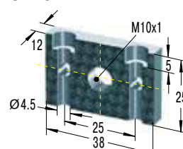
通用转接件
