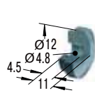
钢冲击头
