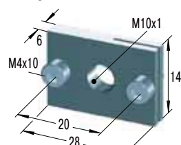
矩形法兰
