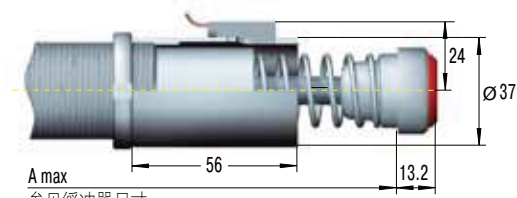
可控限位套筒
