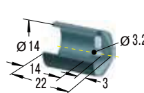
钢套
