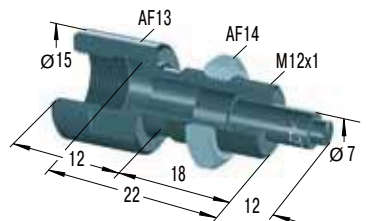
偏心转接器
