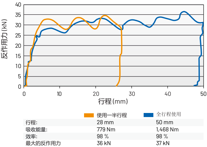
特性曲线 型号 CD-88-53 力-行程 特性曲线
