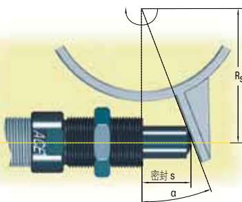
旋转运动行程末端的柔性阻尼
