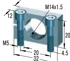
固定支架
