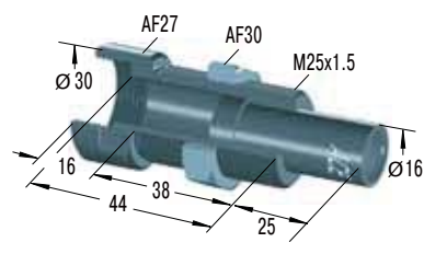
偏心转接器
