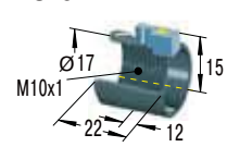
可控限位套筒
