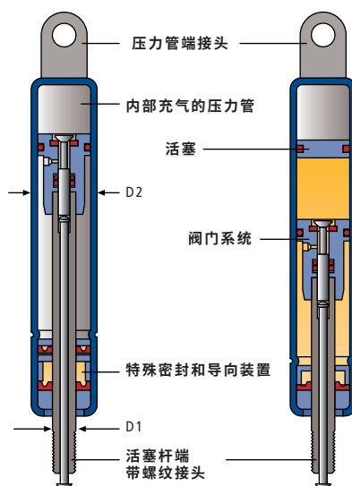
左面:弹性锁止气弹簧 BLOC-O-LIFT®
